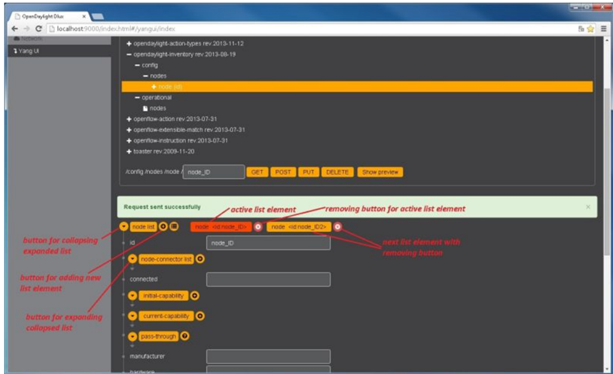
Fig. 1.16: DLUX List Elements
