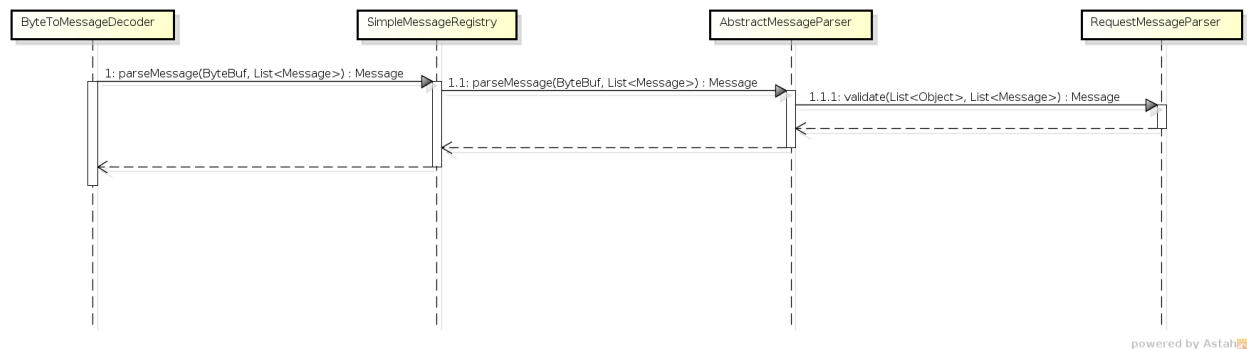
Fig. 2.45: Parsing
