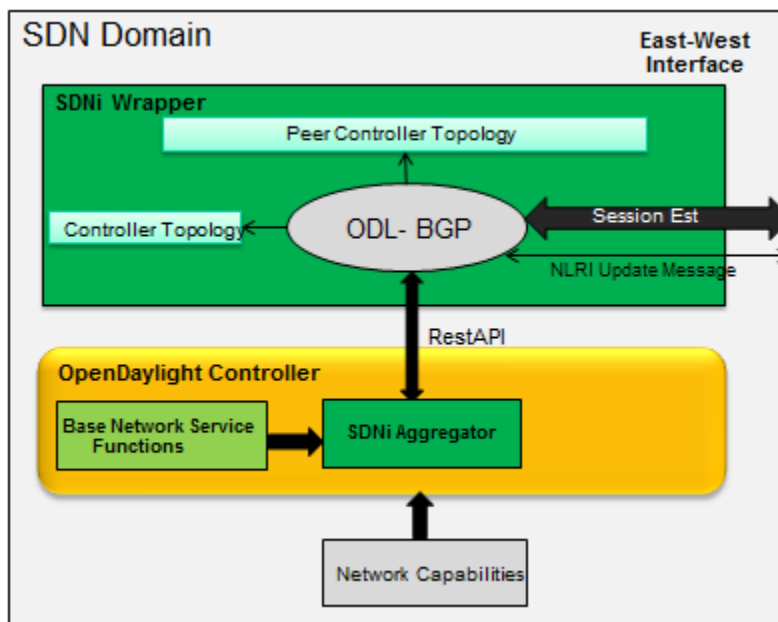
Fig. 2.28: SDNiWrapper
