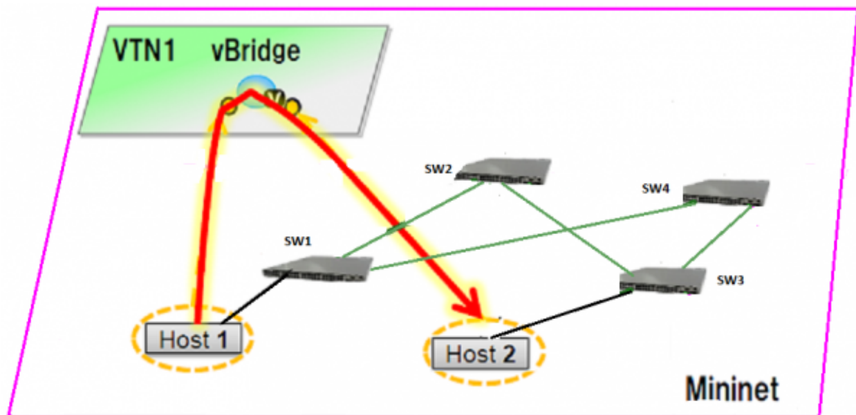
Fig. 1.151: PathMap
