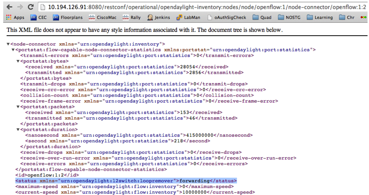
Fig. 1.67: STP status
