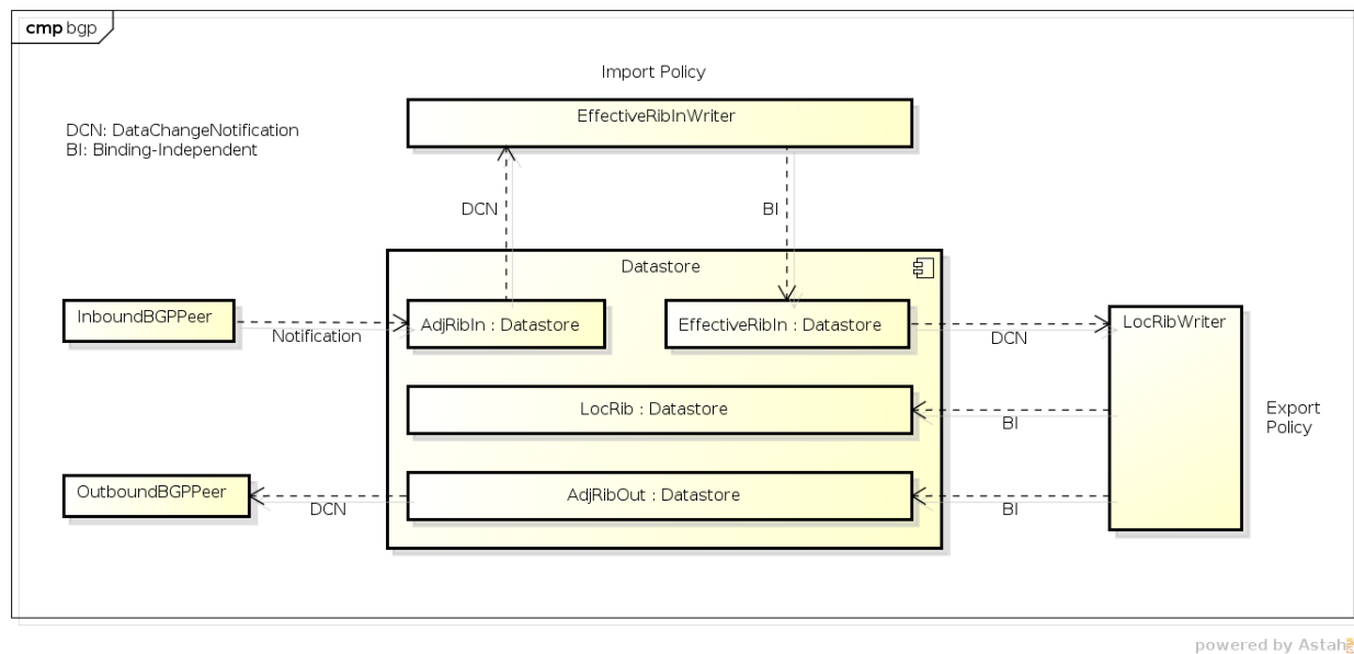
Fig. 2.16: RIB
