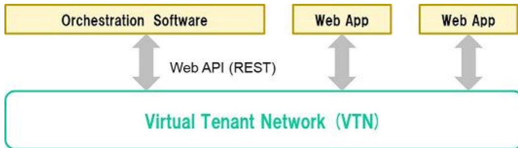
Fig. 1.117: VTN API
